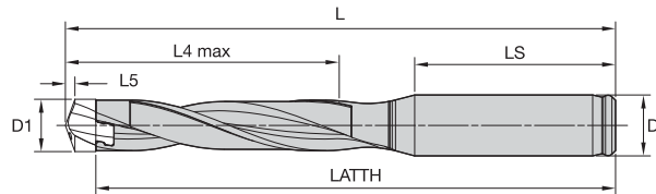
円筒形丸シャンク (SSシャンク)
